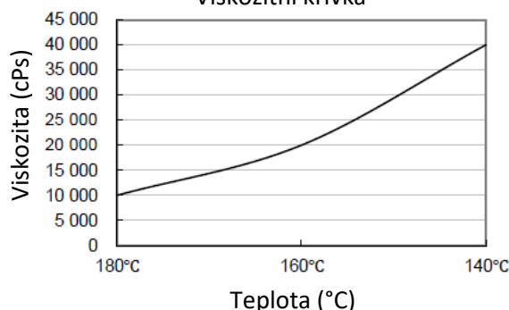
Viskozitní křivka
