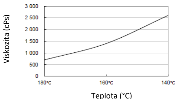
Viskozitní křivka
